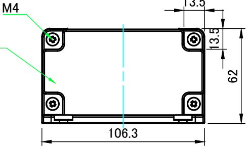
フランジ付側板2 Flanged end panel 2
